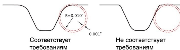
Рисунок 17. Закругленность желобков
