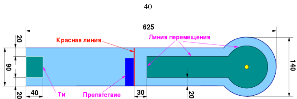
Рисунок 3. Основные размеры и разметка дорожки стандарта «миниатюр-гольф»
