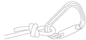
Рисунок 6. Баррел (применяется только для крепления к карабину самостраховки)
